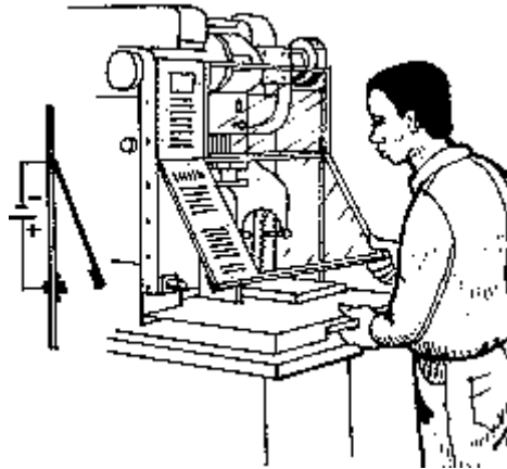
Рисунок 53б. Внешнее защитное приспособление, использующее устройство автоматического отключения
