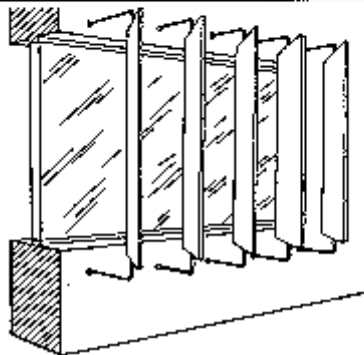
Рисунок 83г. Внешние вертикальные экраны против солнечной радиации. (I) Постоянно зафиксированные.(ii) приспособляемые
